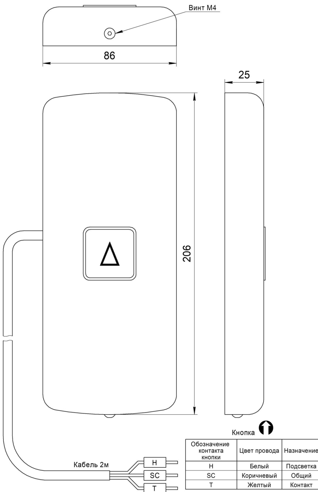
Рис.1 Внешний вид и габаритные размеры Вызывного поста ВП-1001-01
